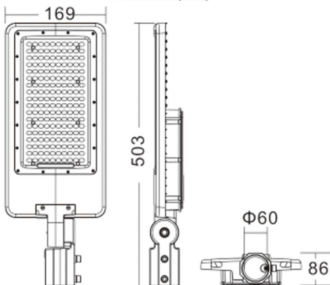
WYMIARY (MM)
